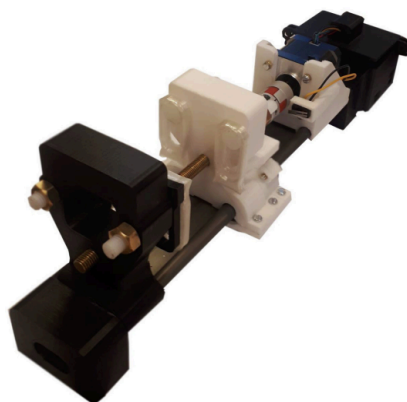
Figura 2. La bomba de jeringa ensamblada, tras la impresión 3D
