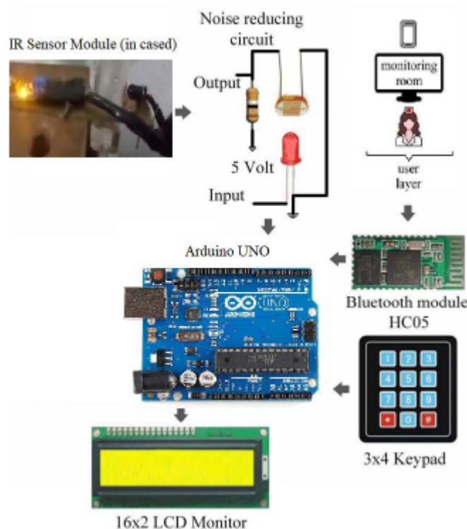
Figura 3. Disposición de los componentes de hardware
